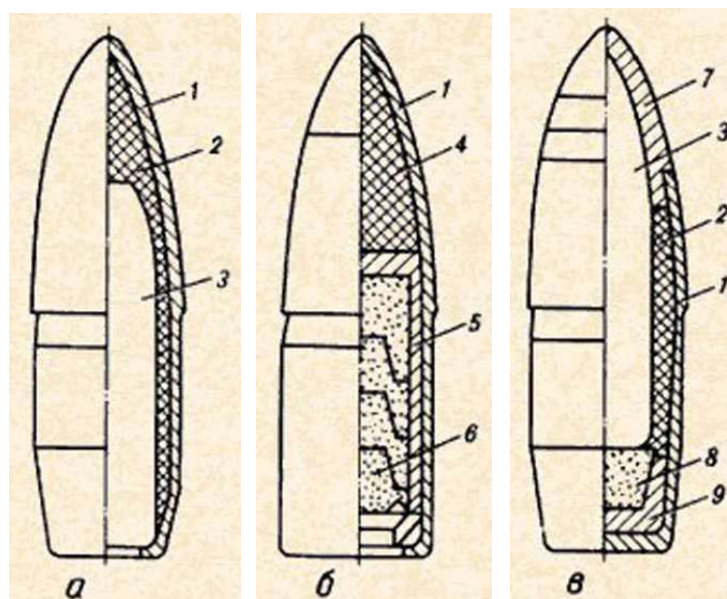
Рис. 49. Пуля: а - обыкновенная со стальным сердечником; б - трассирующая; в - бронебойно-зажигательная; 1 - оболочка; 2 - свинцовая рубашка; 3 - стальной сердечник; 4 - свинцовый сердечник; 5 - стаканчик трассера; 6 - трассирующий состав; 7 - томпаковый наконечник; 8 - зажигательный состав; 9 - свинцовый поддон
