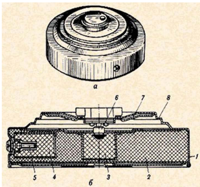
Рис. 13. Противотанковая мина ТМ-57:
