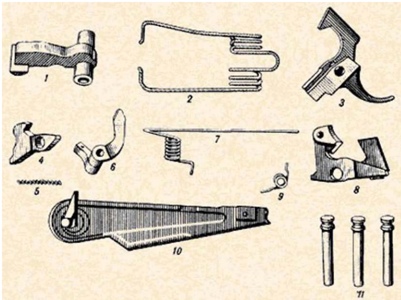
Рис. 35. Ударно-спусковой механизм:
