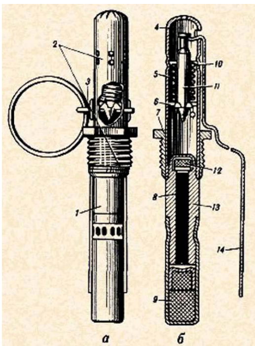
Рис. 73. Запал гранаты УЗРГМ: а - общий вид; б - разрез; 1 - собственно запал; 2 - ударный механизм; 3 - предохранительная чека; 4 - трубка ударного механизма; 5 - боевая пружина; 6 - шайба ударника; 7 - соединительная втулка; 8 - замедлитель; 9 - капсюль-детонатор; 10 - направляющая шайба; 11 - ударник; 12 - капсюль- воспламенитель; 13 - втулка замедлителя; 14 - спусковой рычаг
