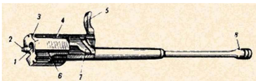
Рис. 31. Затворная рама с газовым поршнем: 1 — канал для затвора; 2 — предохранительный выступ; 3 — выступ для опускания рычага автоспуска; 4 — паз для отгиба ствольной коробки; 5 — рукоятка; б — паз для отражательного выступа; 7 — фигурный вырез; 8 — газовый поршень
