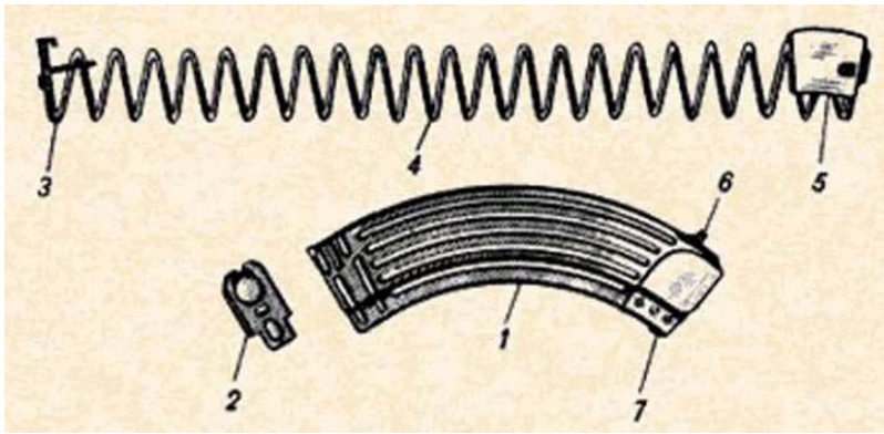
Рис. 37. Магазин:
