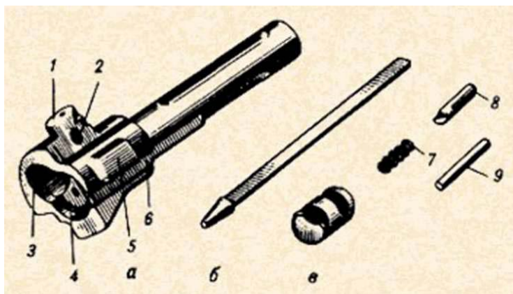
Рис. 32. Затвор:
