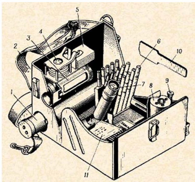
Рис. 126. Войсковой прибор химической разведки (ВПХР):
