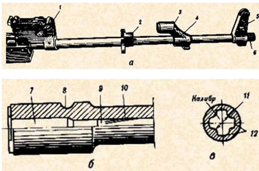
Рис. 27. Ствол:
