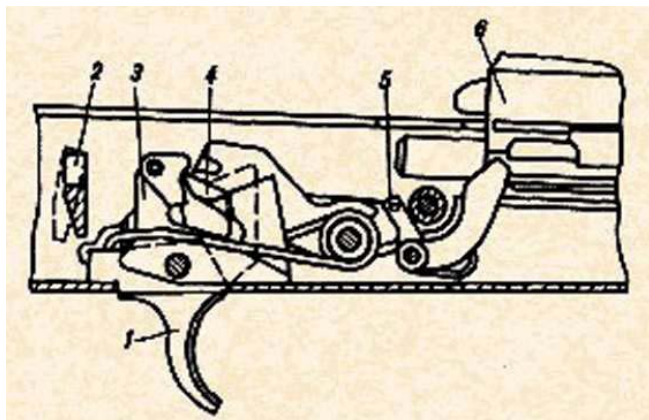
Рис. 52. Положение частей ударно-спускового механизма перед выстрелом:
