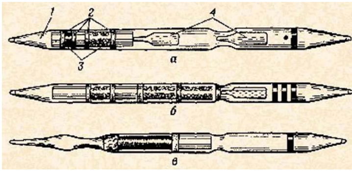
Рис. 127. Индикаторные трубки для определения ОВ: а — зарина и V-газов; б — фосгена, синильной кислоты и хлорциана; в — иприта; 1 — корпус трубки; 2 — ватные тампоны; 3 — накопитель; 4 — ампулы с реактивами
