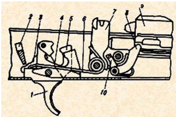
Рис. 51. Положение частей ударно-спускового механизма до заряжания
