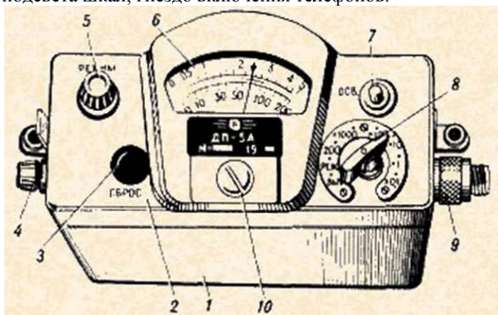
Рис. 122. Измерительный пульт рентгенметра ДП-5А:
