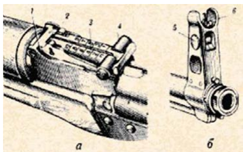
Рис. 30. Прицельное приспособление: а — прицел; б — основание мушки; 1 — колодка прицела; 2 — пластинчатая пружина; 3 — продольная планка; 4 — хомутик; 5 — полозок с мушкой; 6 — предохранитель мушки
