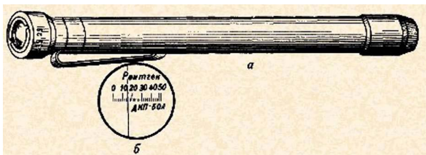
Рис. 125. Дозиметр ДКП-50А: а - общий вид; б – шкала
