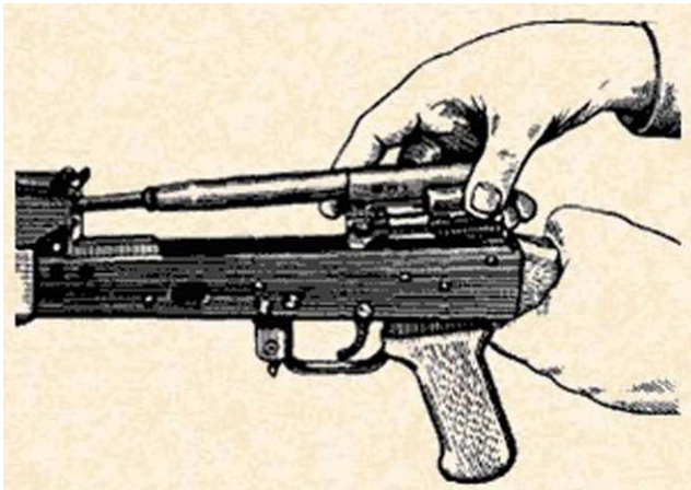
Рис. 44. Отделение затворной рамы с затвором.
