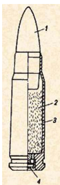
Рис. 48. Боевой патрон; 1 - пуля; 2 - пороховой заряд; 3 - гильза; 4 - капсюль
