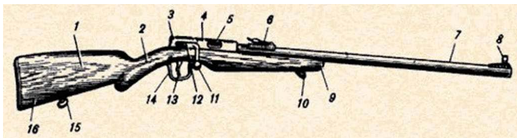
Рис. 58. Малокалиберная винтовка ТОЗ-8:
