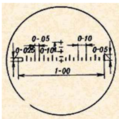
Рис. 63. Угломерные шкалы бинокля
