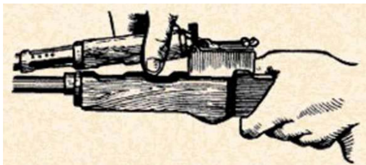
Рис. 46. Отделение газовой трубки со ствольной накладкой.
