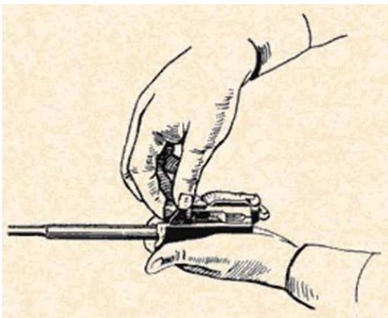
Рис. 45. Отделение затвора от затворной рамы
