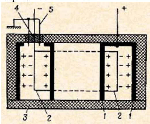
Рис. 118. Схема ионизационной камеры:
