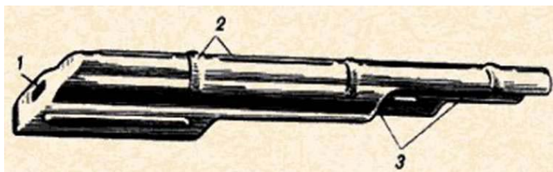
Рис. 29. Крышка ствольной коробки: 1 — отверстие; 2 — ребра жесткости; 3 — ступенчатые вырезы
