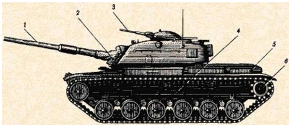
Рис. 9. Уязвимые места танка: 1 — ствол пушки; 2 — приборы стрельбы и наблюдения; 3 — ствол пулемета; 4 — борт корпуса; 5 — корма корпуса; 6 — ходовая часть
