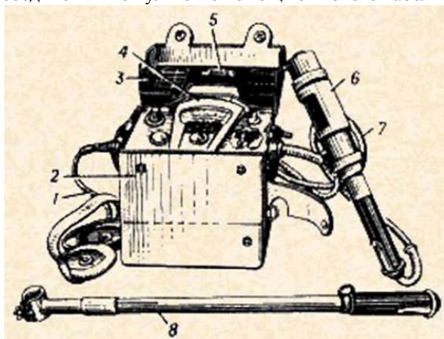
Рис. 121. Рентгенметр ДП-5А: 1 — кабель телефонов; 2 — футляр; 3 — крышка футляра; 4 — измерительный пульт; 5 — контрольный препарат; 6 — зонд; 7 — кабель зонда; 8 — удлинительная штанга
