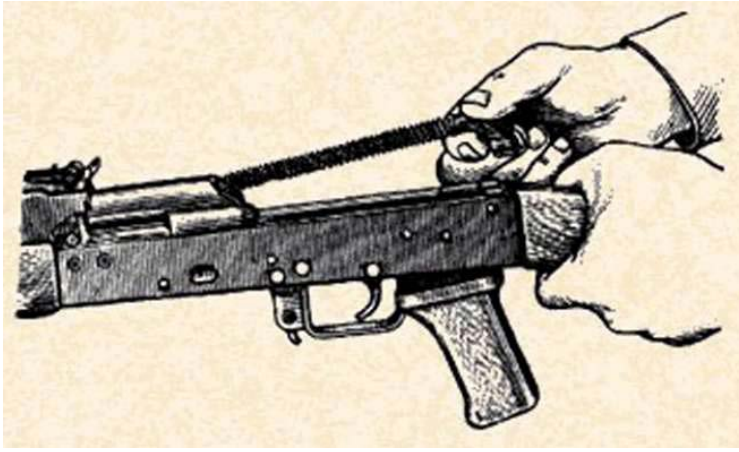
Рис. 43. Отделение возвратного механизма
