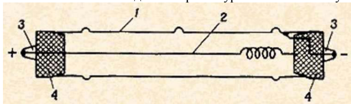
Рис. 120. Газоразрядный счетчик с металлическим корпусом: 1 — корпус счетчика (катод); 2 — нить счетчика (анод); 3 — выводы; 4 — изоляторы
