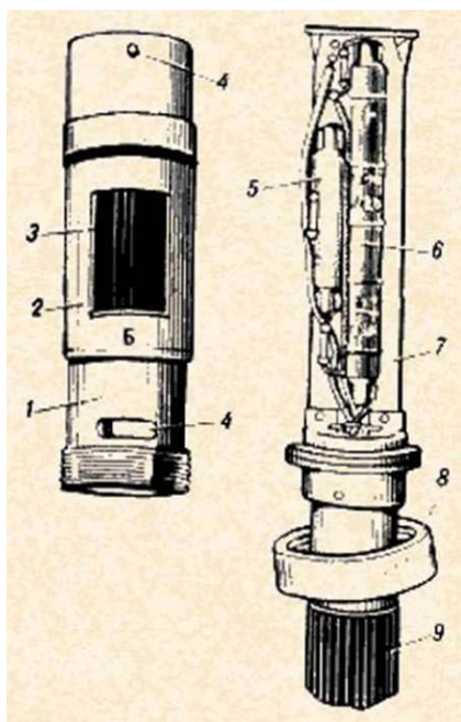
Рис. 123. Зонд со снятым корпусом:
