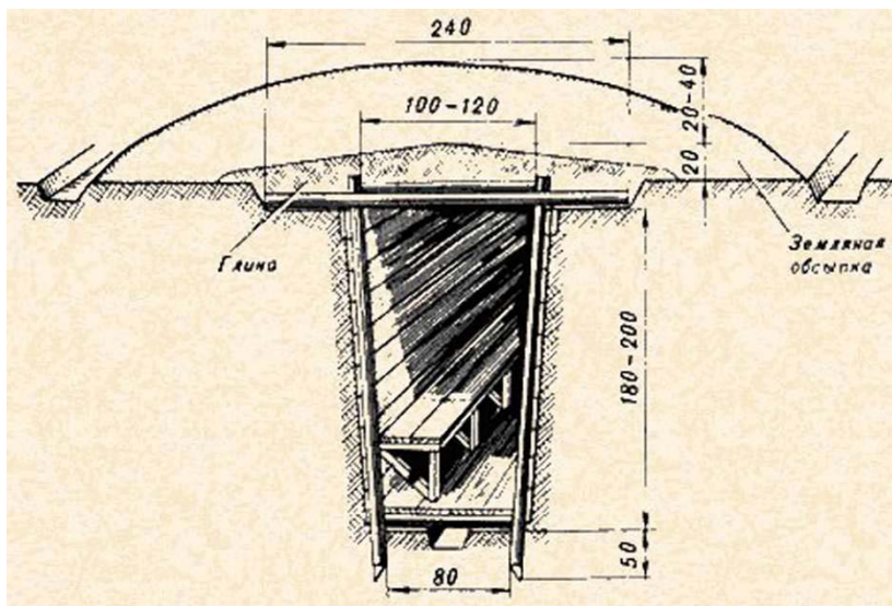
Рис. 116. Перекрытая щель (размеры даны в сантиметрах)
