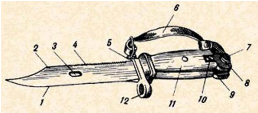
Рис. 38. Штык-нож:
