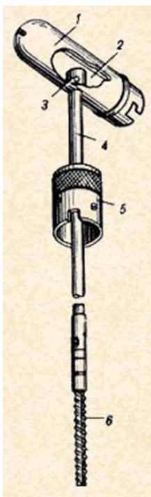
Рис. 56. Принадлежность автомата, подготовленная для чистки: 1 — пенал; 2 — отвертка; 3 — головка шомпола; 4 — шомпол; 5 — крышка пенала; 6 — протирка.
